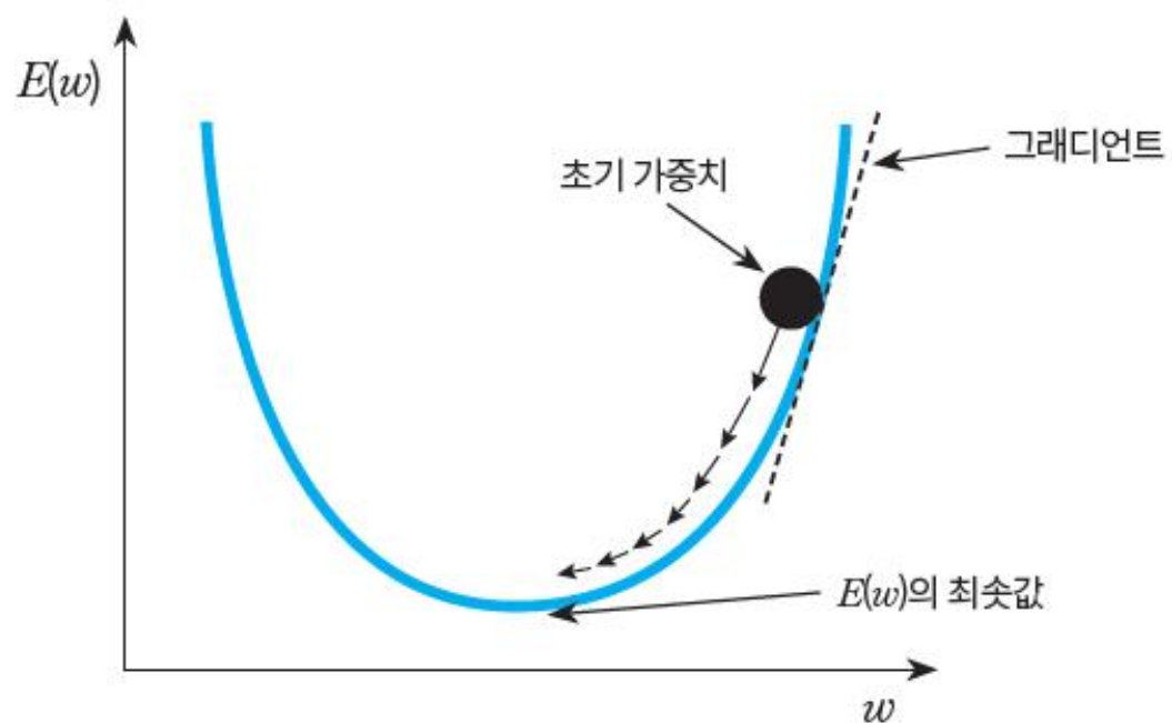
그림 10-8 경사하강법
