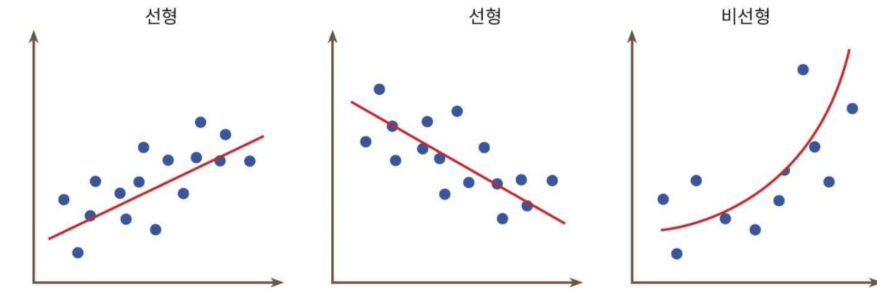
그림 10-1 회귀의 종류
